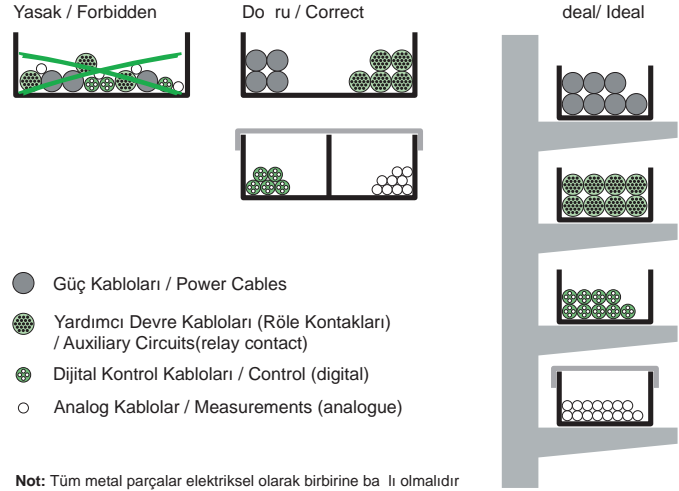
Şekil 3. Grup halinde kablolar için kablo kanalına önerilen dşşeme şekli Fig.3:Recommendation of installation of groups of cables on cable trays
